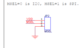
SPI/I2C SEL
