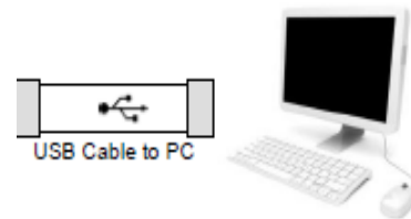
IDE Tools
